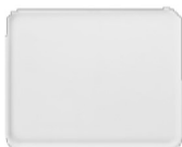
VASSOIO PORCELLANA BIANCA SMALTATA CODICE DIMENSIONE EV-202627 175*325xh15mm, GN 1/3 EV- 202628 354*325xh15mm, GN 2/3 EV- 202629 265*325xh15mm, GN 1/2
