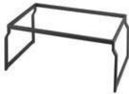
RISER GN 1/1 DRITTO LIV. 2 ACCIAIO INOX VERNICIATO A POLVERE CODICE DIMENSIONE 19938-003 530*325*253 mm, GN 1/1
