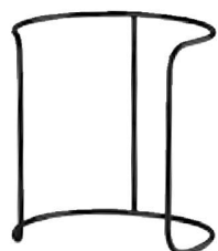
SUPP. TONDO ALTO NERO ACCIAIO INOX 18/10 NERO OPACO CODICE DIMENSIONE EV-230746 ø 250xh260 mm
