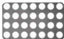
INSERTO YOGURT I/1 IN PLEXIGLASS 28 FORI DA 55 MM CODICE DIMENSIONE EV-YOGB 530*325 mm, GN 1/1
